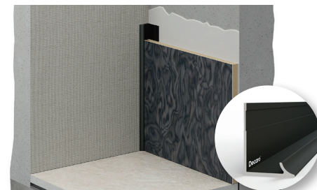
Оформление внутреннего угла 90 с помощью углового внутреннего профиля D1184
