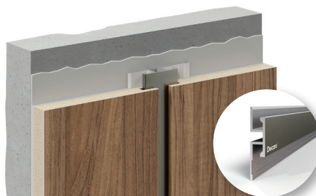
Прямая стыковка панелей с помощью соединительного профиля D1187
