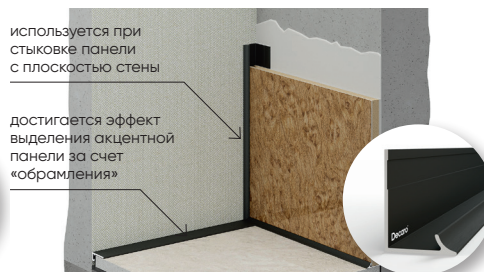
Оформление внутреннего угла 90 с помощью углового внутреннего профиля D1184 и микроплнтуса M15
